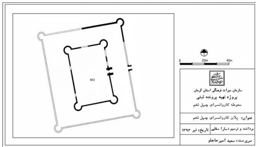
نقشه ۱۴. نقشه ساختارهای برجای مانده از کاروانسرای چهل تخم
