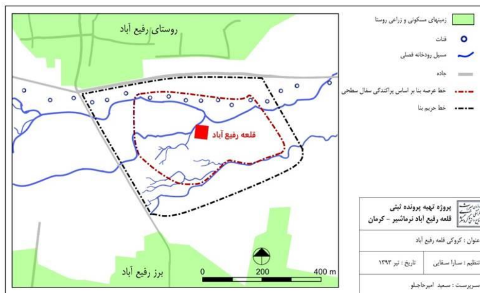
نقشه ۹. کروکی محل قلعه رفیع آباد
