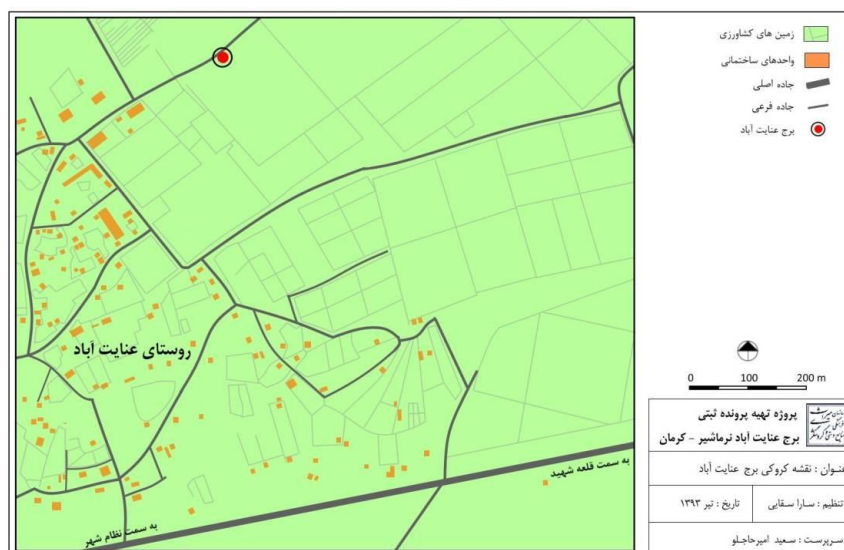
نقشه ۱۲. کروکی برج عنایت‌آباد در میانه باغات و نخلستان‌های روستای عنایت‌آباد
