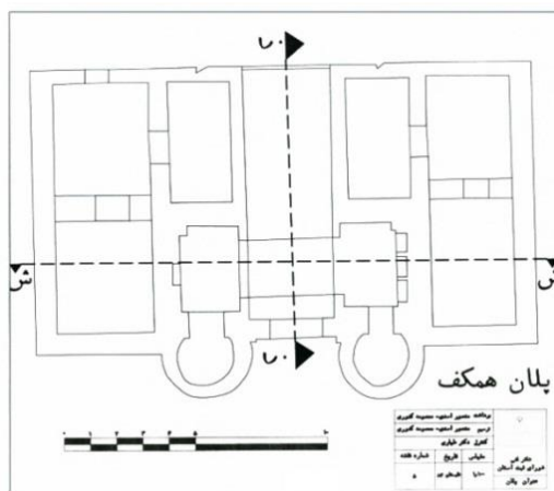
نقشه ۱۱. نقشه طبقه همکف از ساختارهای برجای مانده از قلعه شهید (شوشی، زاده، ۱۳۸۴: ۱۱)
