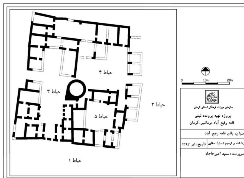
نقشه ۱۰. پلان قلعه رفیع آباد
