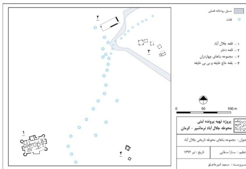
نقشه ۵. مجموعه بناهای محوطه جلال‌آباد
