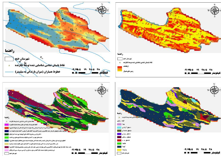
شکل ۶ وضعیت شاخص‌های خطوط بارش، ناهمواری‌ها، زمین‌شناسی و شکل زمین (مأخذ: نگارندگان، ۱۳۹۸)
