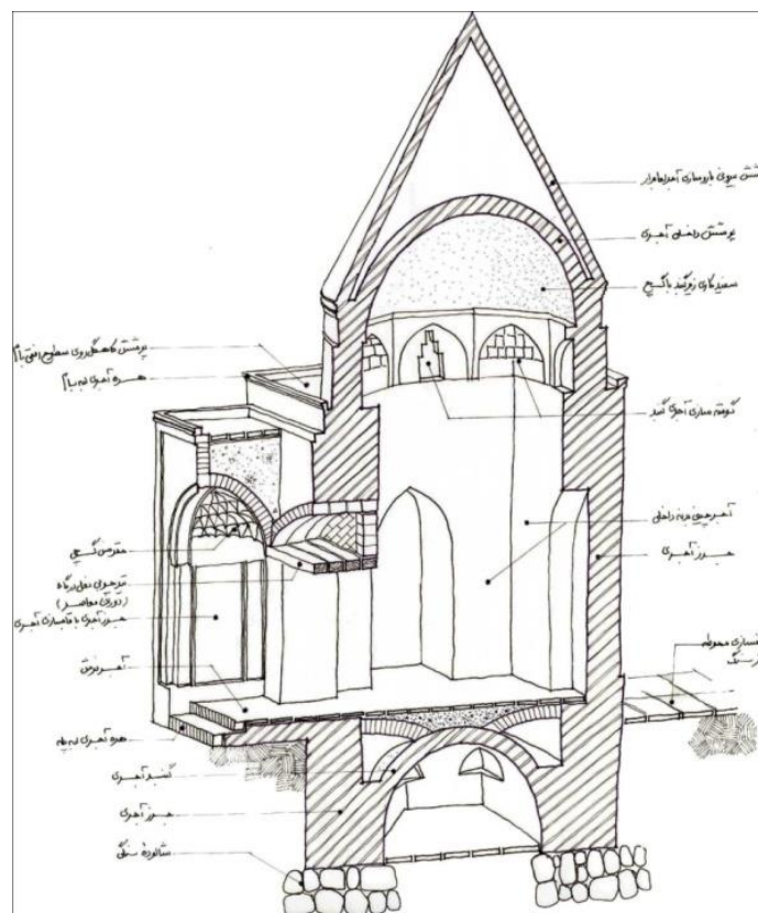
تصویر ۳۳: نمایش سه بعدی عناصر سازه‌ای و تزئینی گنبد غازان‌خان و نحوه‌ی ارتباط آنها (زندیکان، ۱۳۸۷/۱: ۶۰)
